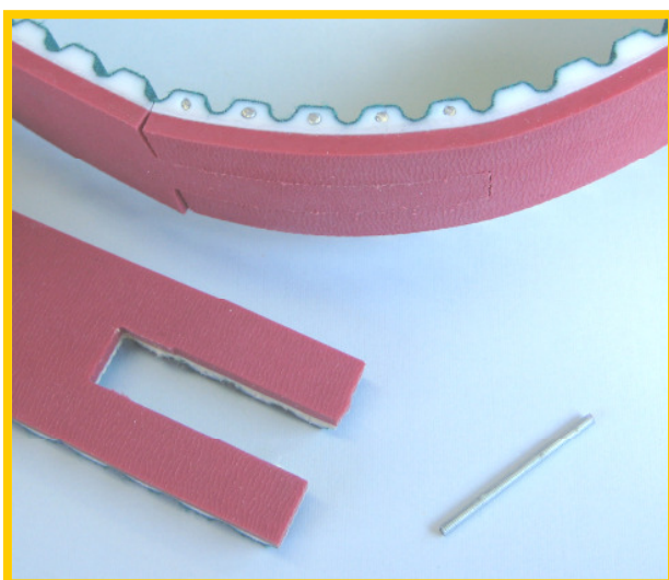
ANSICHT: ZAHNSEITE
