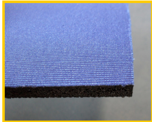
TYP FBA SCHWARZ MIT NYLON OFFENZELLIG MAX. DICKE: 6MM HÄRTER ALS TYP S
